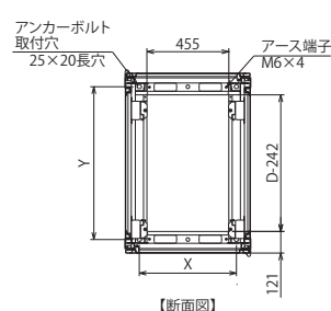
【断面図】
