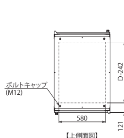
【上側面図】
