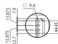
C部詳細 (拡大)
