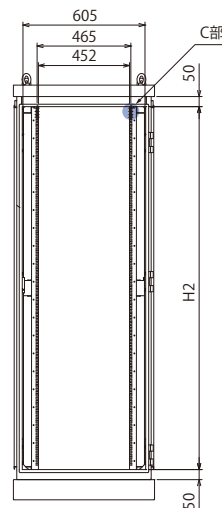
ドアを取外した状態
