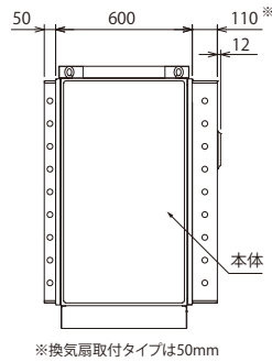
断面A-A 電子クーラータイプ
