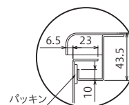
F部断面図
