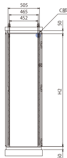
ドアを取外した状態
