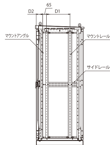
A-A断面
