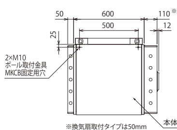
断面A-A 電子クーラータイプ
