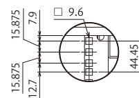
C部詳細 (拡大)
