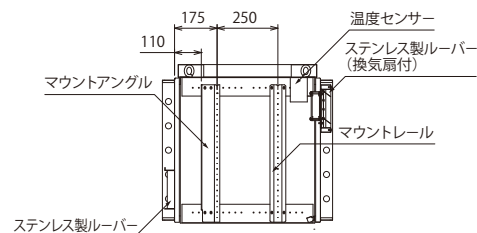
断面A-A 換気扇取付タイプ
