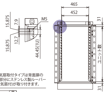
扉を外した状態 (正面図)
