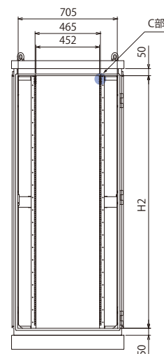
ドアを取外した状態
