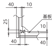
基板取付金具図
