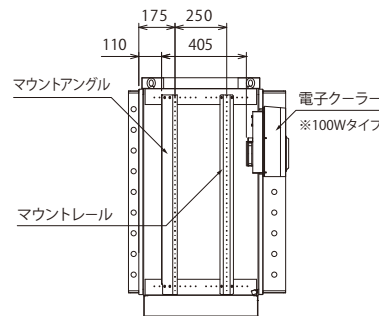
断面A-A 電子クーラータイプ
