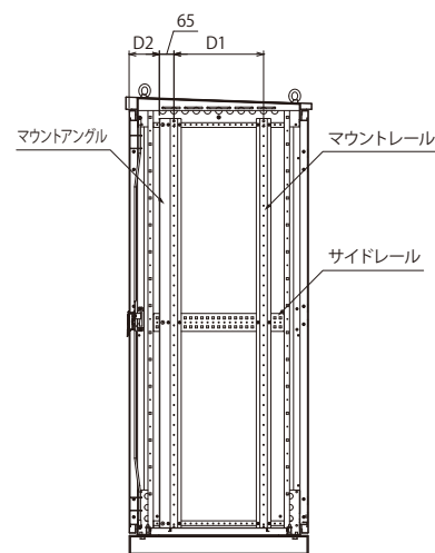
A-A断面
