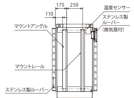
断面A-A 換気扇取付タイプ
