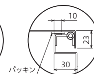
G部断面図
