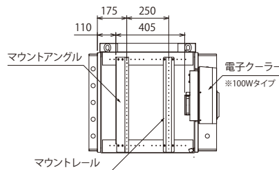
断面A-A 電子クーラータイプ
