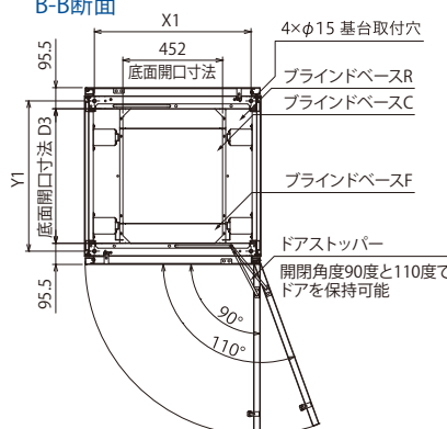
B-B断面
