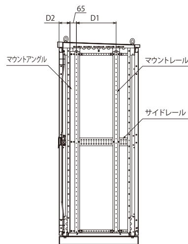
A-A断面
