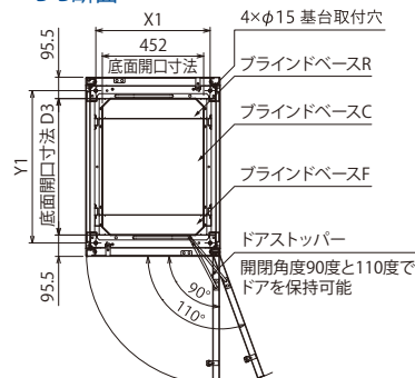
B-B断面
