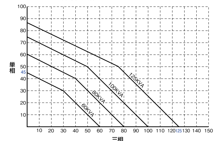
●トランスの負荷分担曲線
