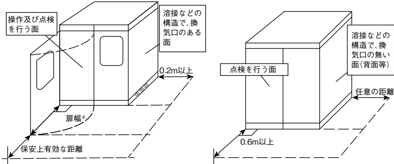
1130－4図 屋内に施設するキュービクルの保有距離
