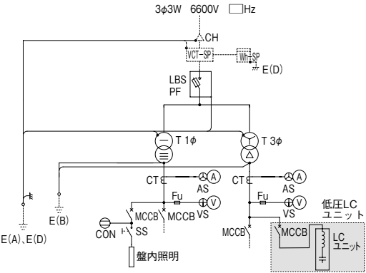
結線図(参考)
