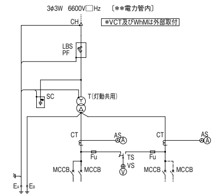
●結線図
