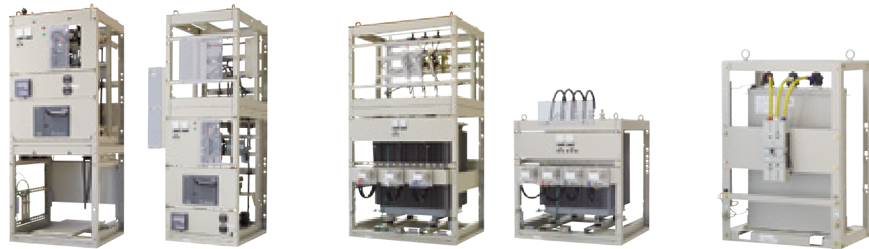
VCB受電盤
