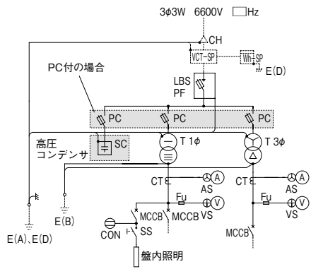
結線図(参考)
