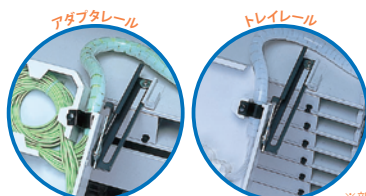
光配線盤
