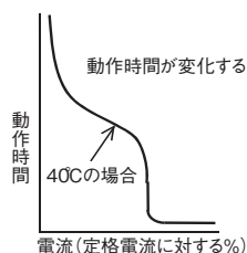
図b 温度補正曲線(例)
