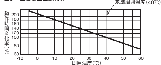
図b 温度補正曲線(例)
