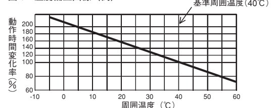
図b 温度補正曲線(例)
