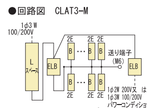
太陽光電池側 ブレーカ
