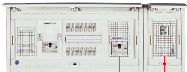
太陽光電池側 ブレーカ 計測ユニット電源用 ブレーカ
