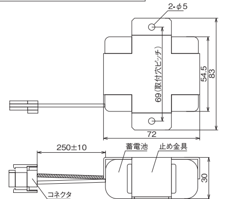
蓄電池および止め金具外形寸法
