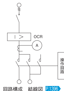
回路構成 結線図 P.1396
