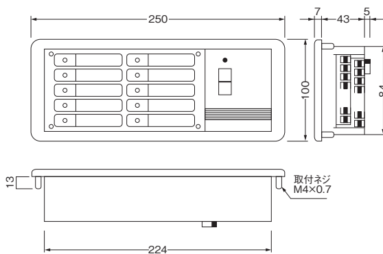
寸法図
